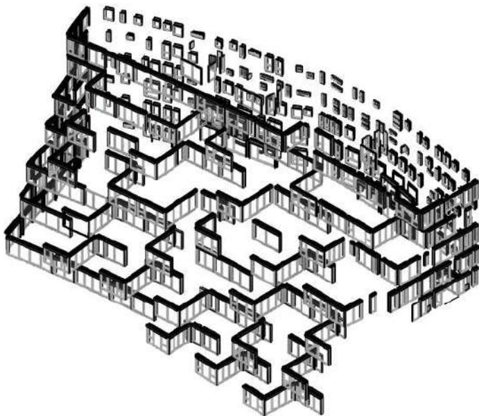
modello BIM dell'edificio con inserimento dei serramenti
