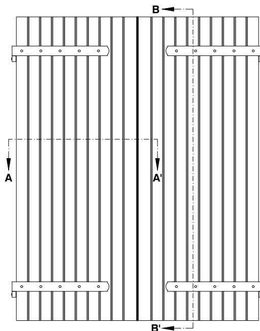
VISTA ESTERNA scala 1:20
