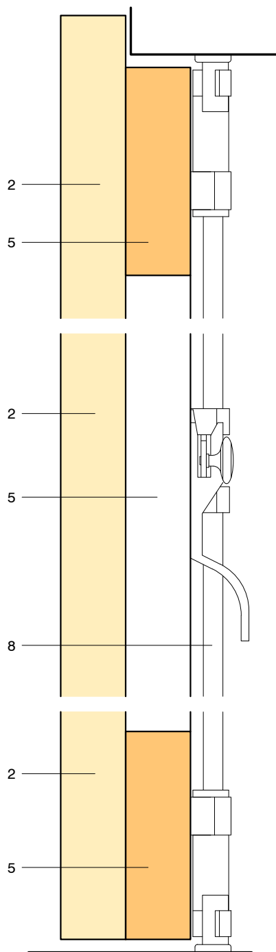
B-B' scala 1:2
