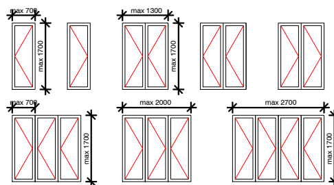
LIMITI DIMENSIONALI APERTURE PREVISTE Destinazioni d'uso UNI 11173 allegato n.3
