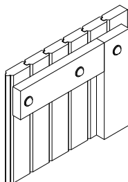
PARTICOLARE ASSEMBLAGGIO
