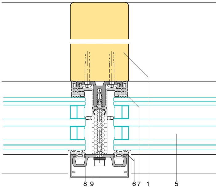
B-B' scale 1:2
