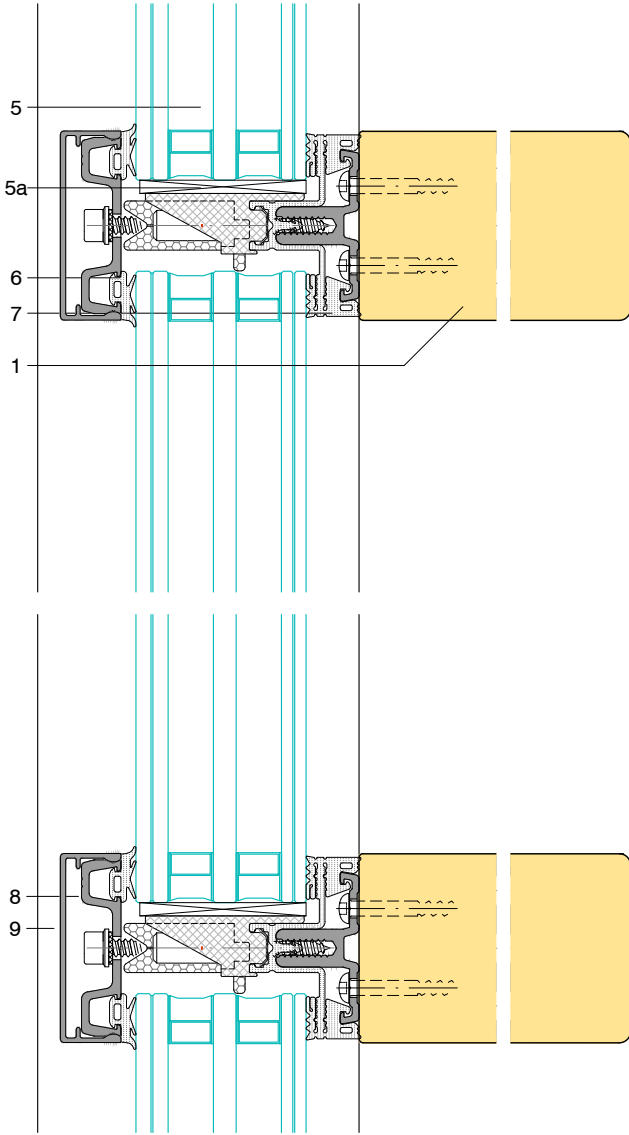
B-B' scale 1:2
